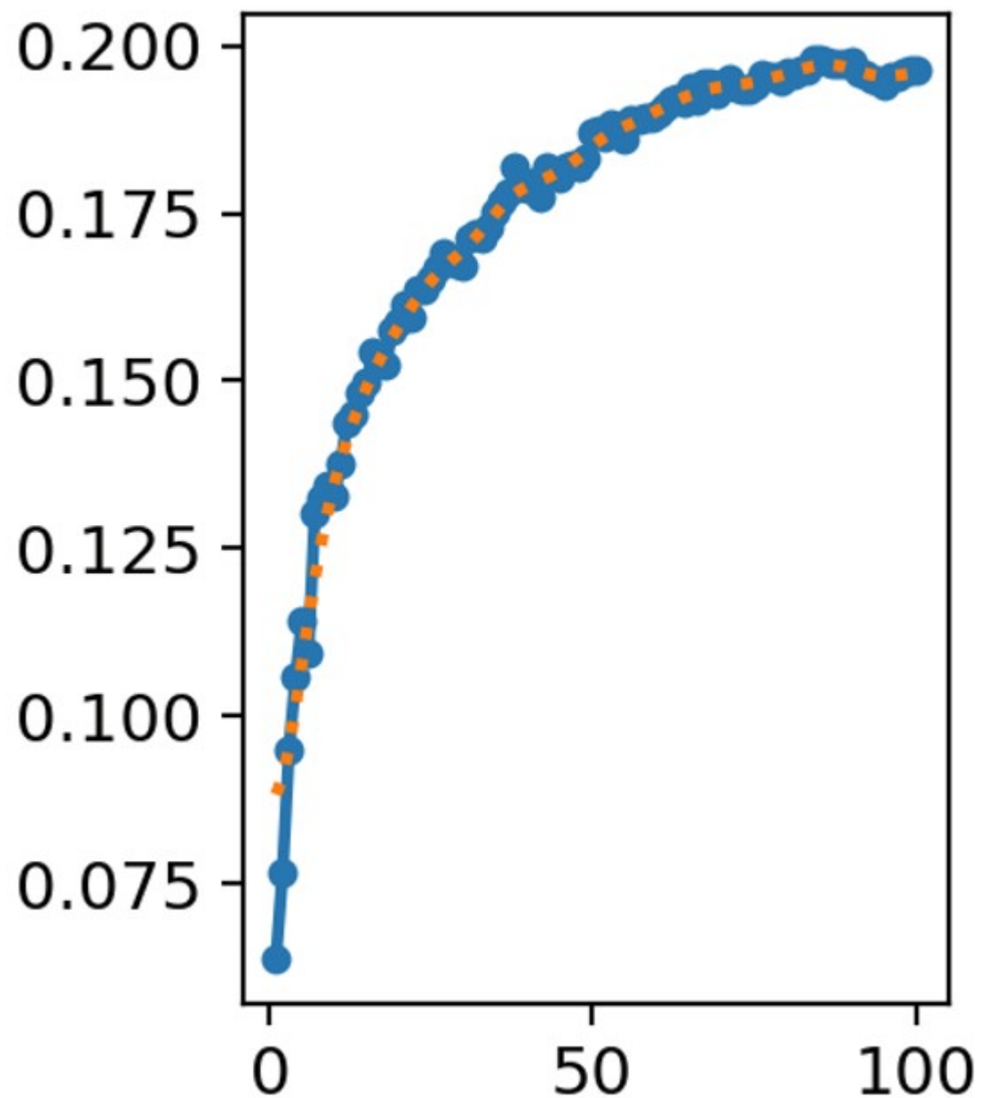
metrics/mAP50-95(B)
